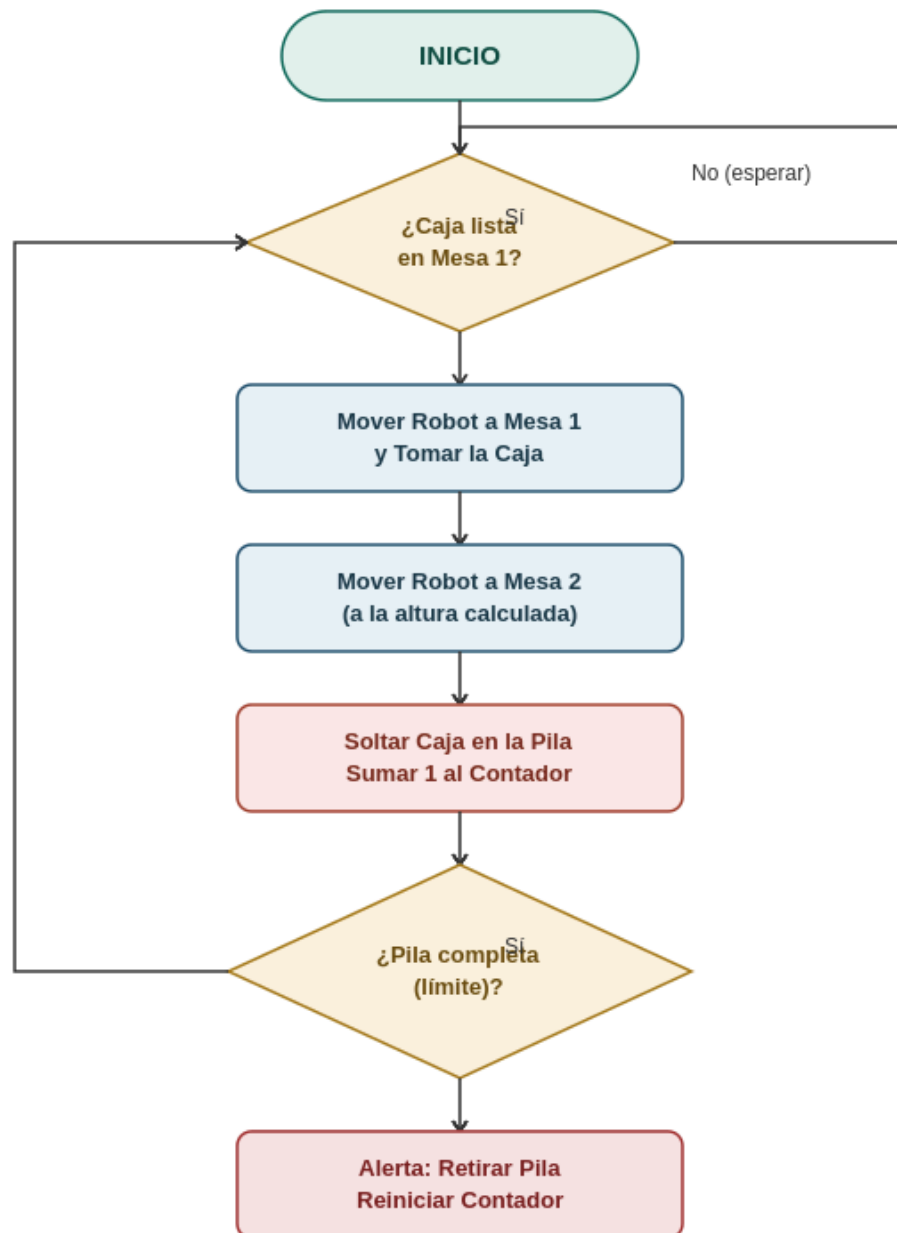
Figura 2. Diagrama de flujo del ciclo de recogida y apilado.
